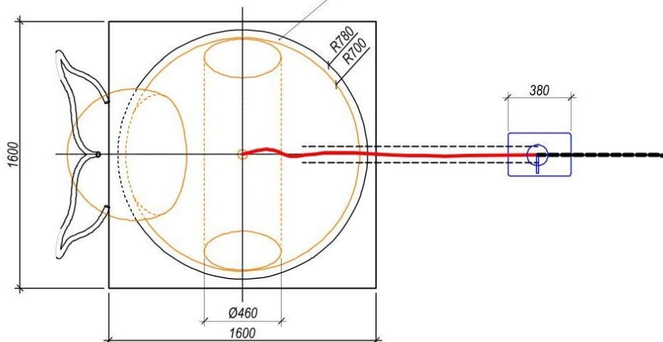
PŮDORYS ZÁKLADU (1:25)
